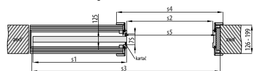
Nákr. 5. PD1P.125 rozsah regulace 125-199mm
